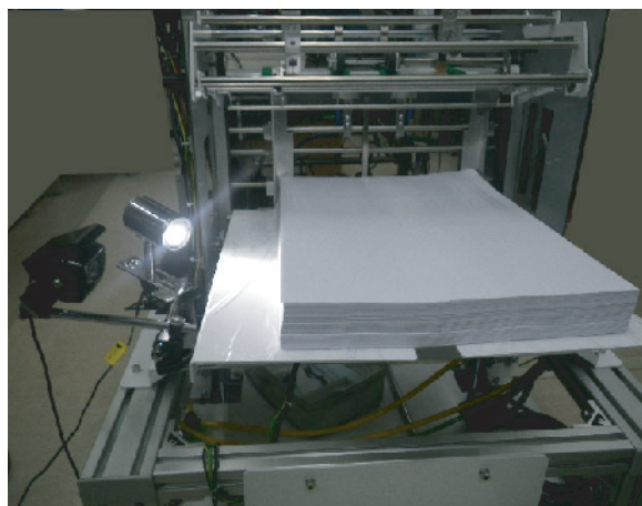
給紙部設置例
